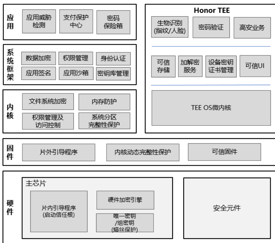
Magic UI 安全架构
